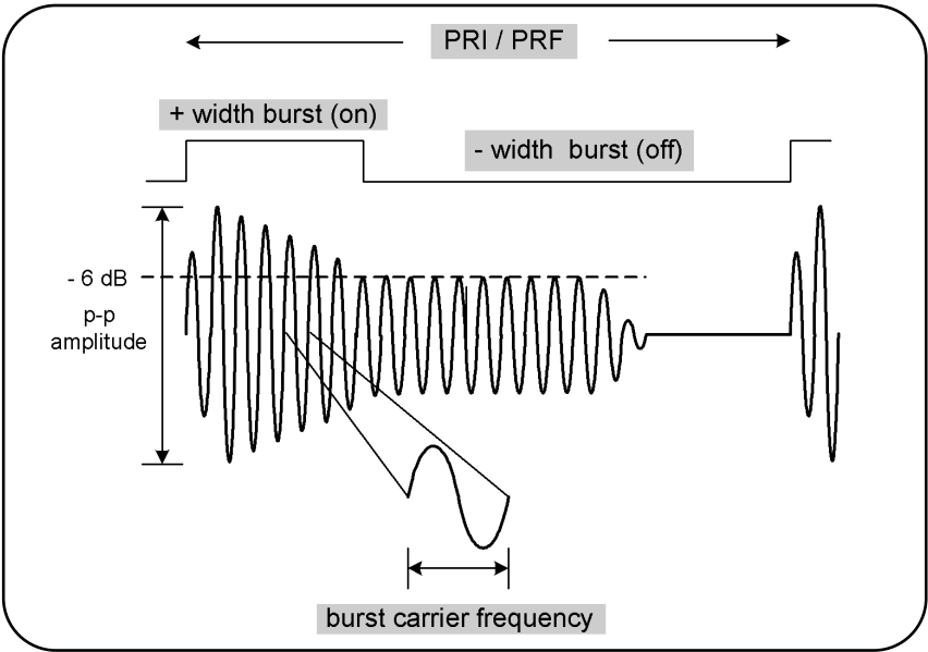
그림 3-13. 53230A의 마이크로 펄스 측정
